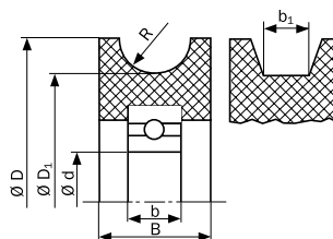
Ausführung ohne Achse (Prinzipskizze)
