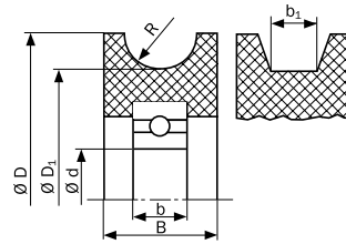
Ausführung ohne Achse (Prinzipskizze)
